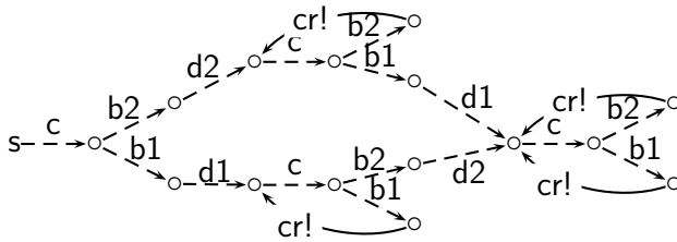
Fig. 14. VMvd \sqsubseteq_{BC} VM2
